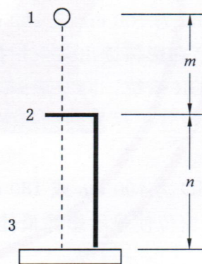
图 3 有效焦点测量示意图
