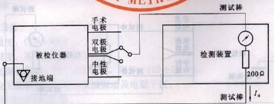
图4 双极电极的高频漏电流
