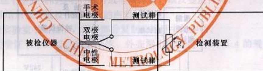
图6 双极模式输出功率测量
