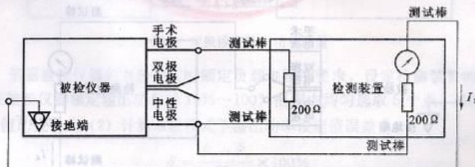
图 1 中性电极以地为基准的高频漏电流
