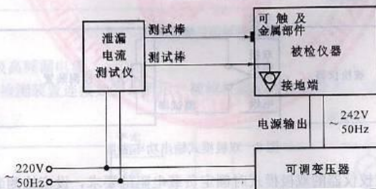
图7 外壳漏电流测量
